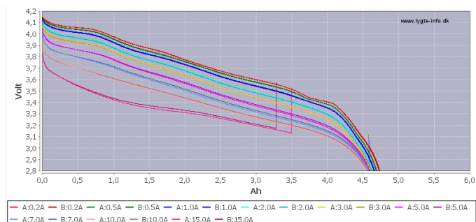
Charakterystyka rozładowania akumulatora : KP ICR21700-500PCM 5000mAh
