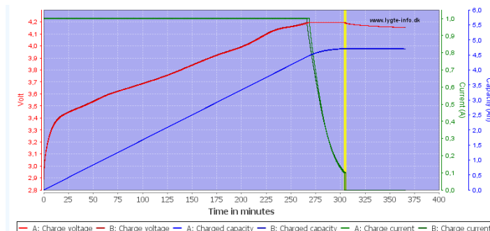
Charakterystyka ładowania akumulatora : KP ICR21700-500PCM 5000mAh
